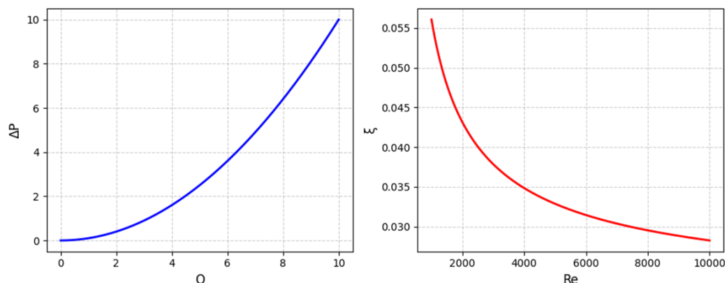
Рис. 1. Давление-поток и гидравлические характеристики
