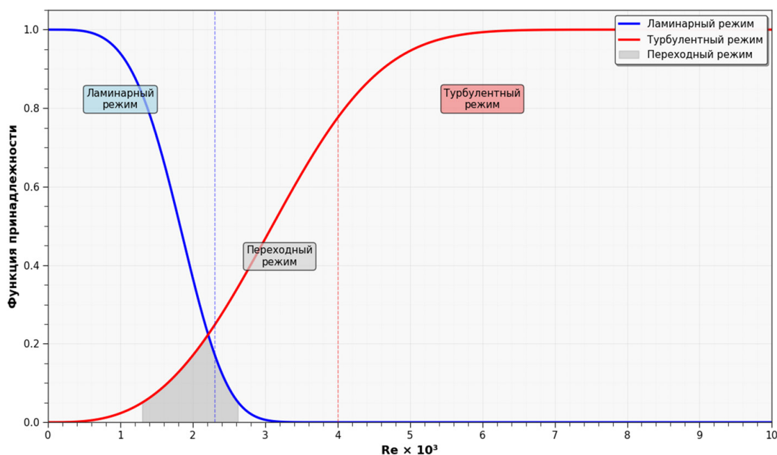
Рис. 4. Функции принадлежности для чёткого множества «Ламинарный режим» и нечётких множеств «Переходный режим» и «Турбулентный режим»
