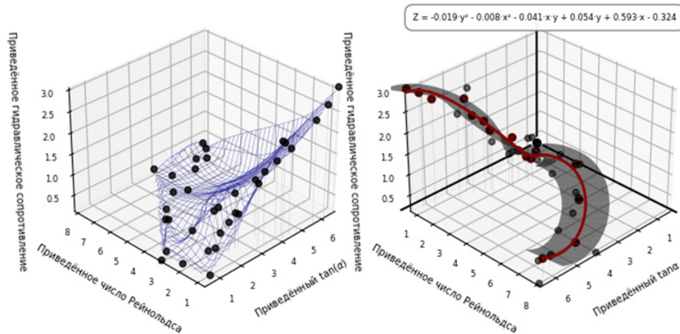
Рис. 4. Трёхмерное представление в системе приведённых координат
