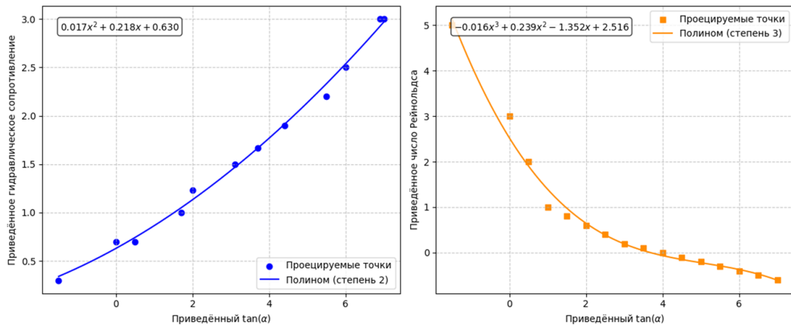
Рис. 5. Графики функций \xi_{\text{пр}} = f(tg \alpha_{\text{пр}}) и Re_{\text{пр}} = f(tg \alpha_{\text{пр}}) в проекции на координатные оси
